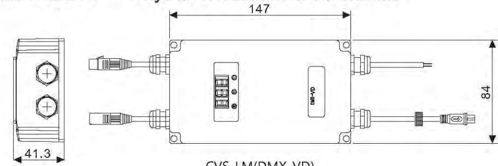
CVS-LM(DMX-VD) 单位/Unit : mm
